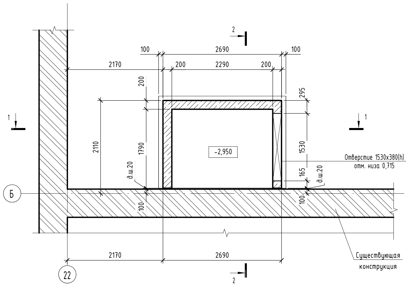
Схема расположения формашты в/о 22-23/Б
