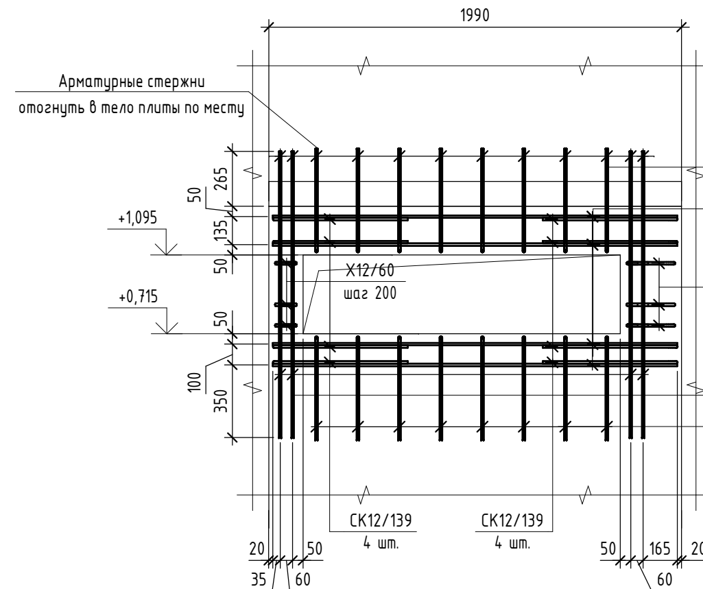
Схема обрамления отверстия в стене
