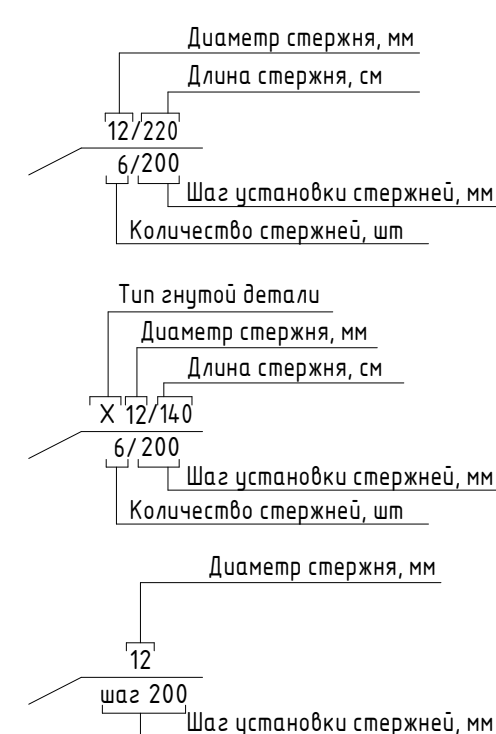
Маркировка позиций арматуры
