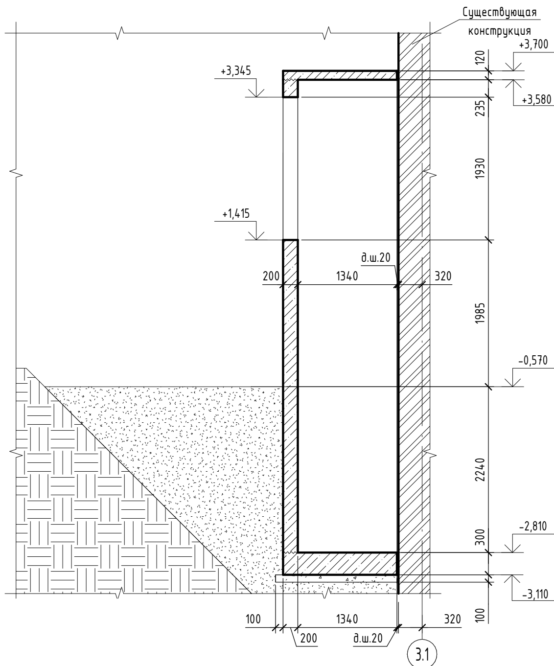
2-2 Опалубка
