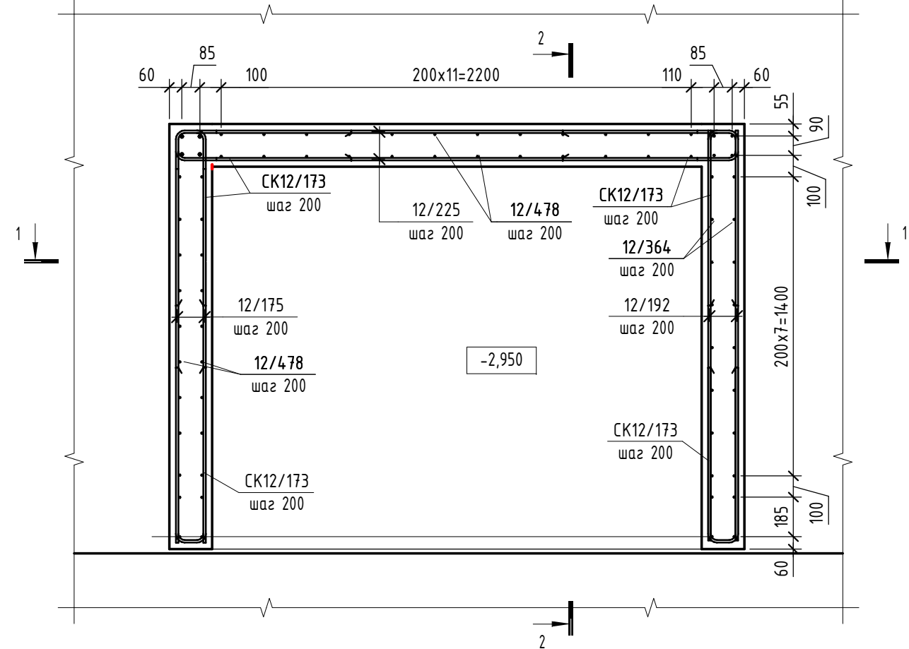
Схема армирования стен формашты в/о 22-23/Б
