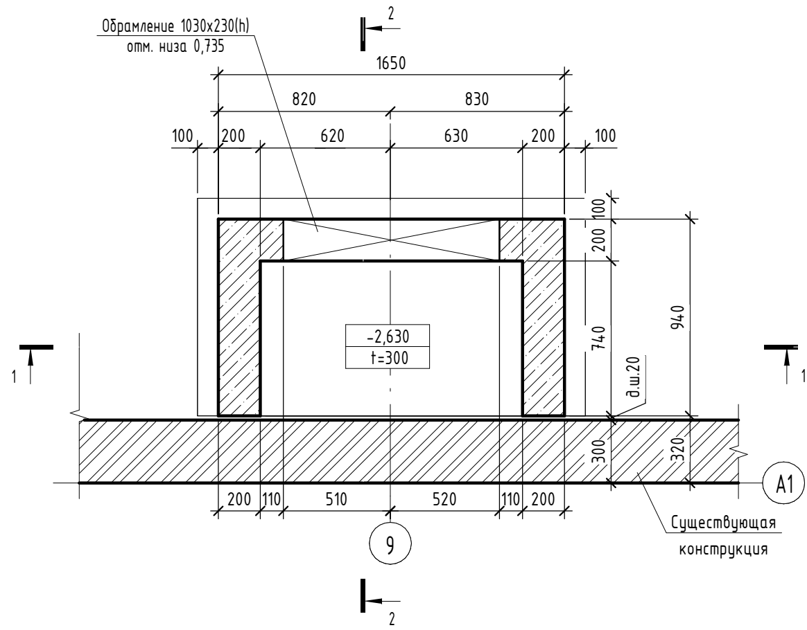
Схема расположения форшахты в/о 9-А1
