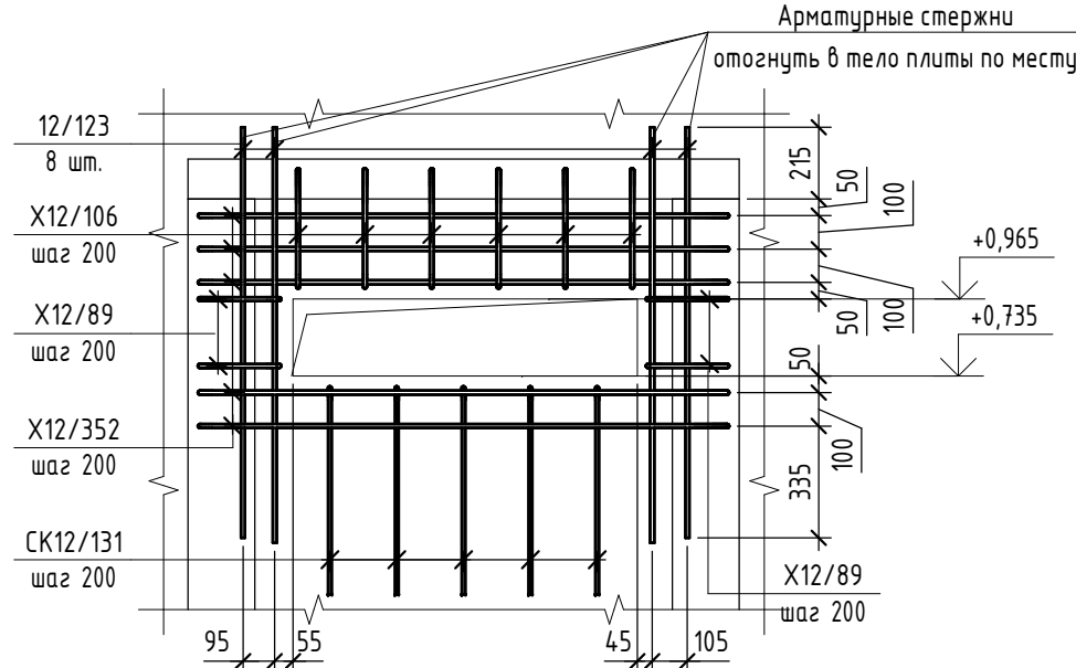
Схема обрамления отверстия в стене
