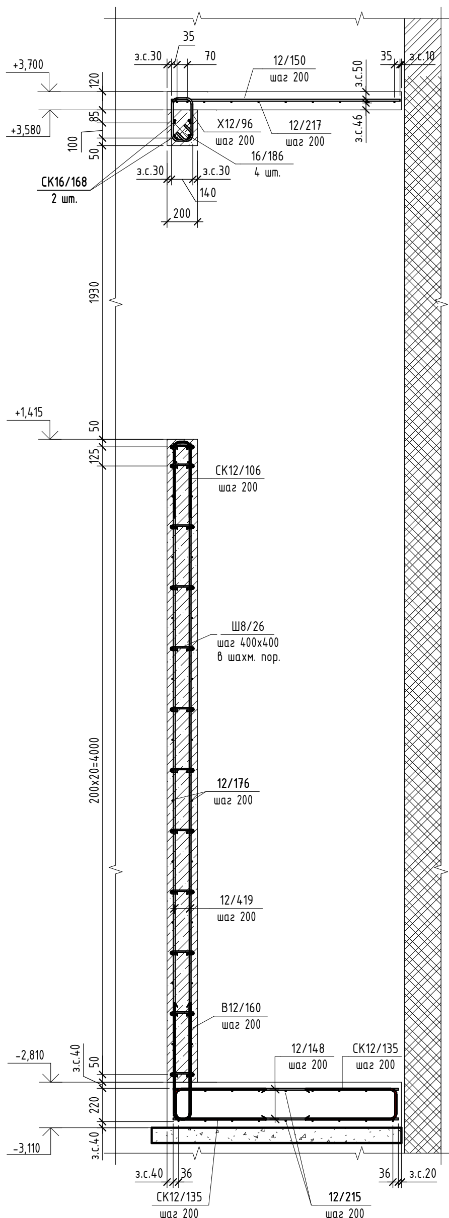
2-2 Армирование
