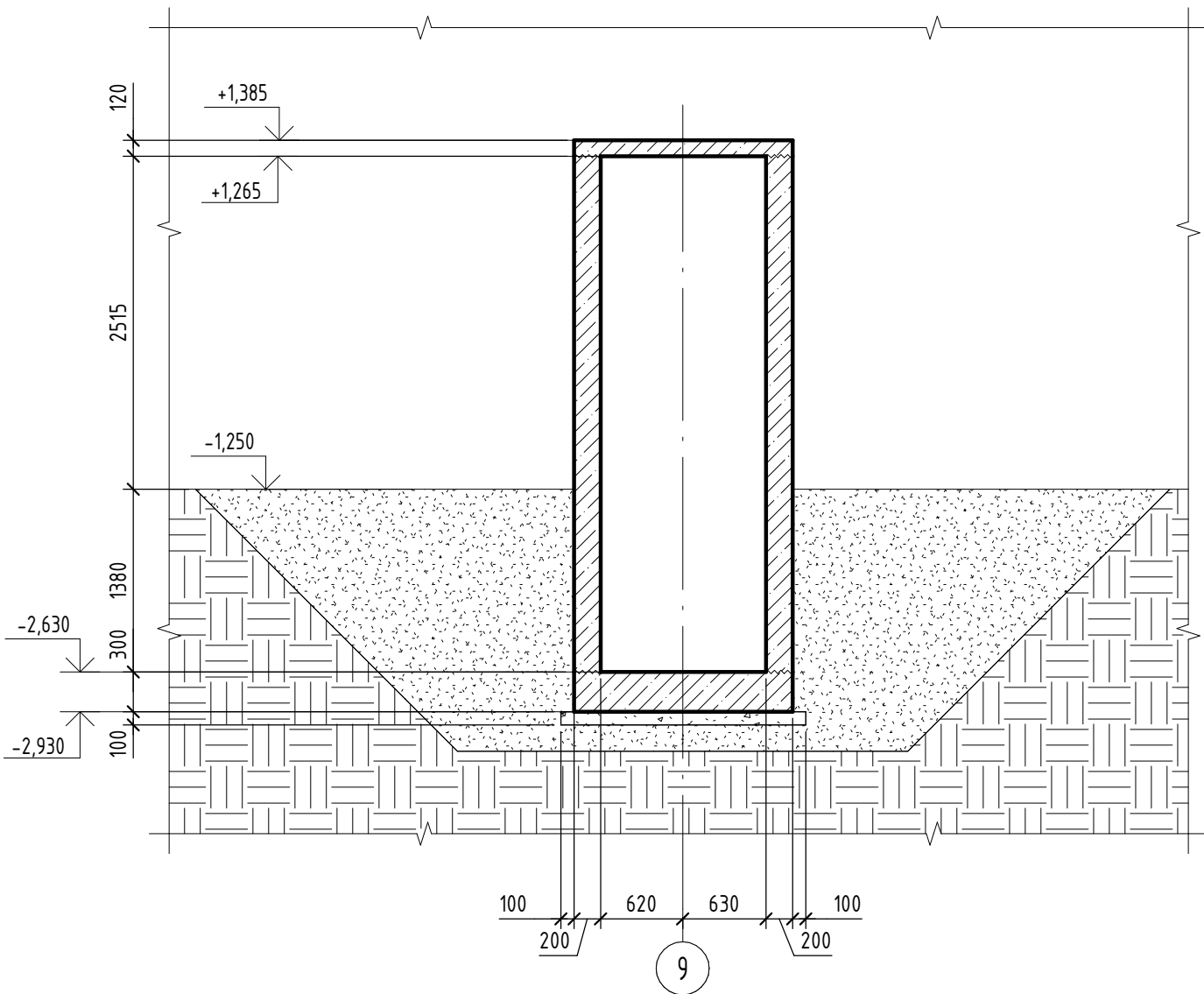
1-1 Опалубка
