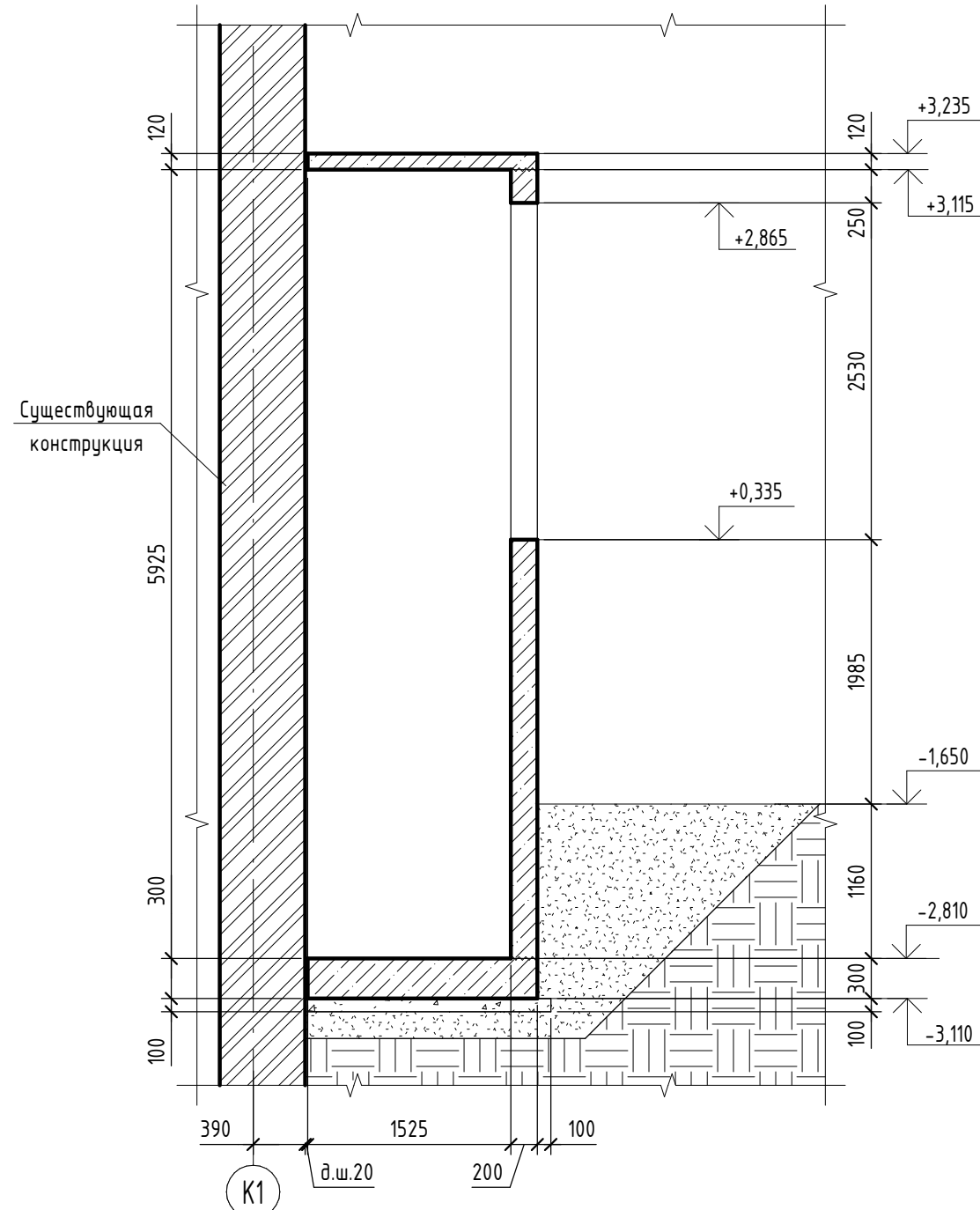
2-2 Опалудка
