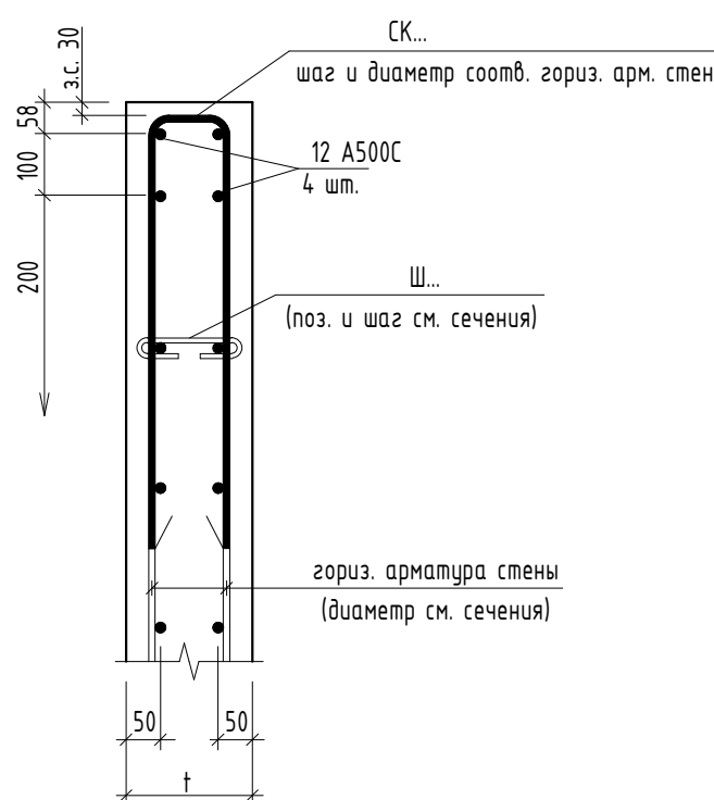
Типовой торцевой узел расположения арматурных стержней
