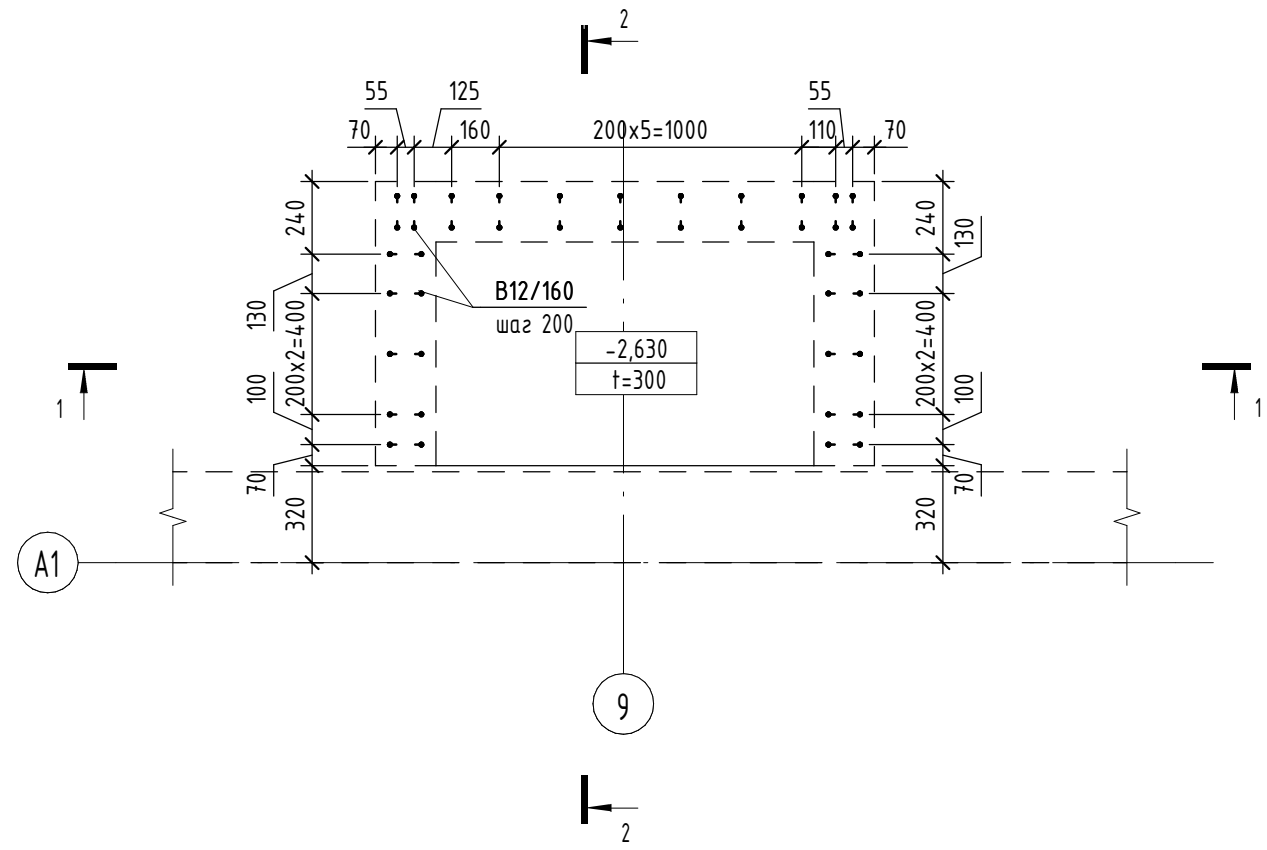
Схема расположения арматурных выпусков вундаментной плиты в/о 9-А1
