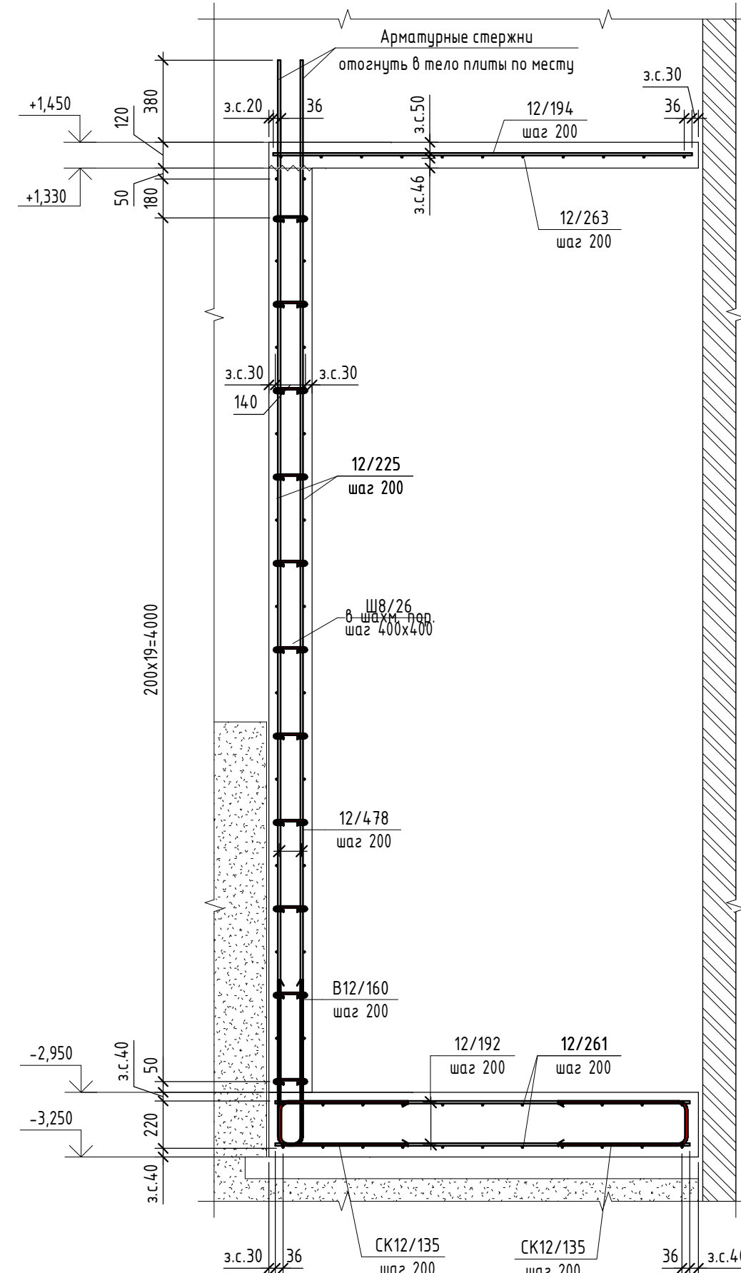
2-2 Армирование
