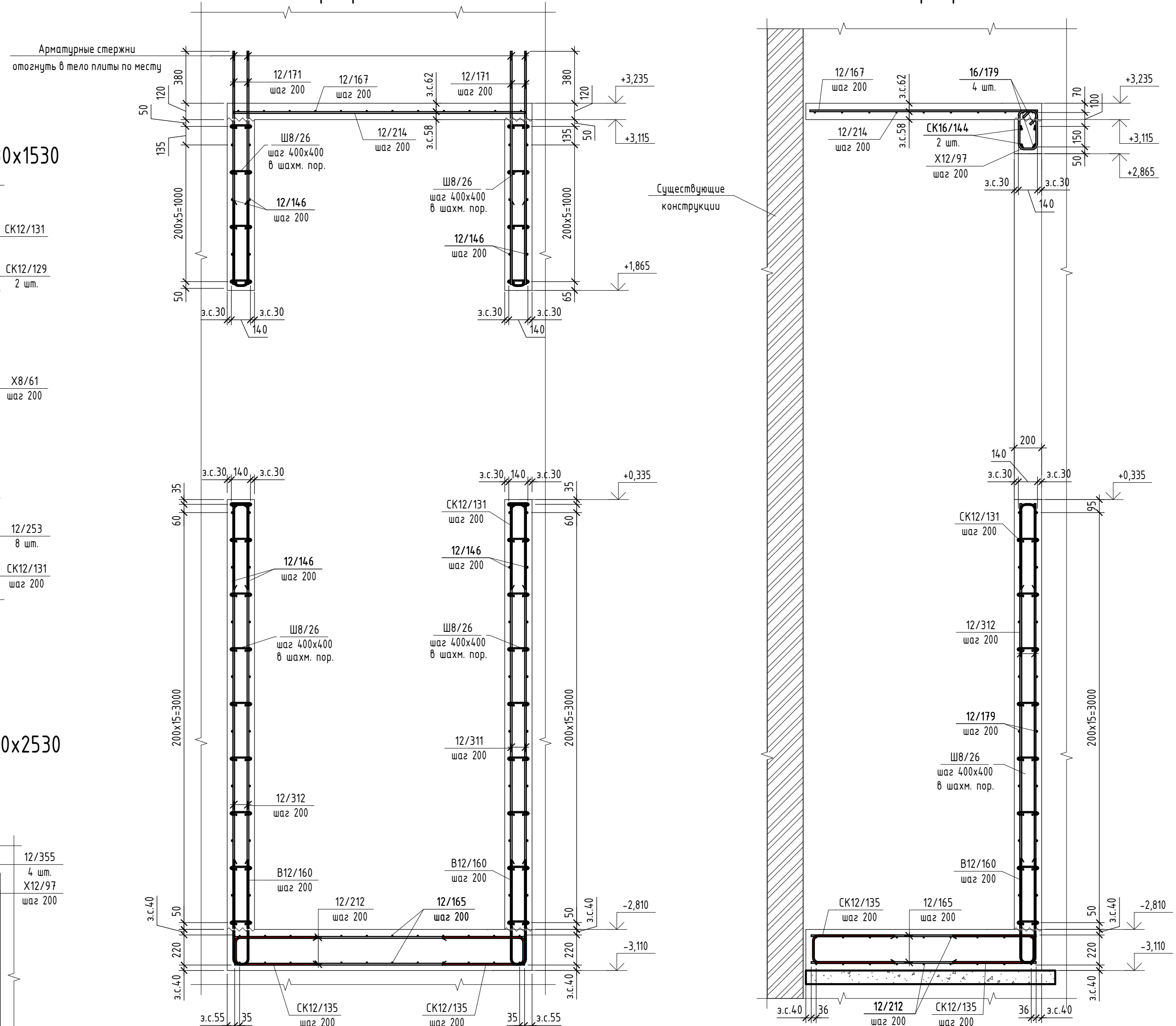
2-2 Армирование
