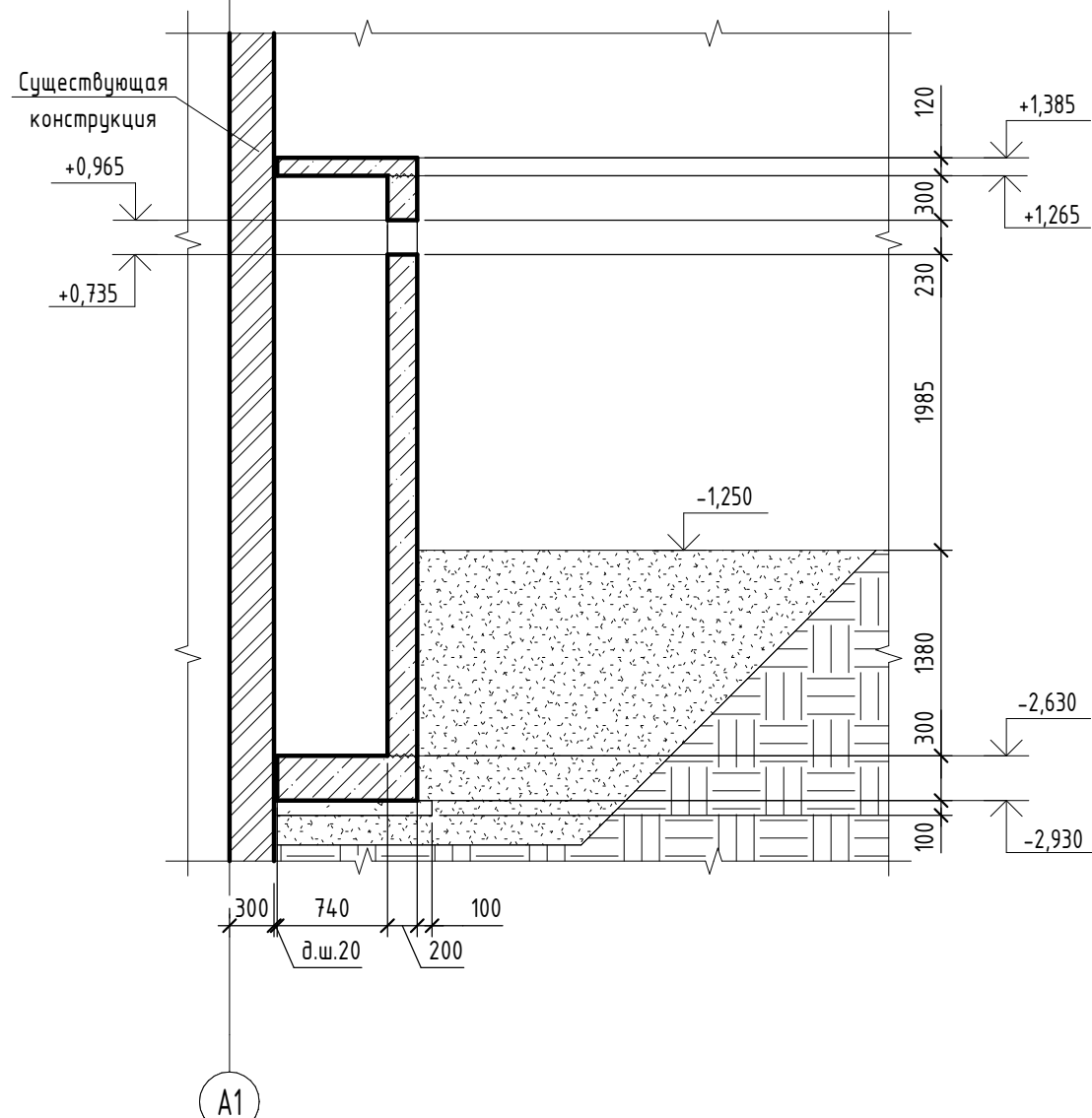
2-2 Опалубка
