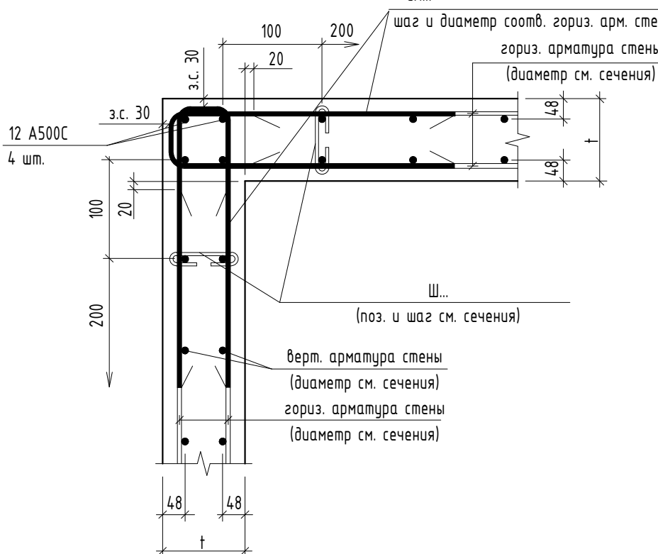
Типовой Г-образный узел расположения арматурных стержней
