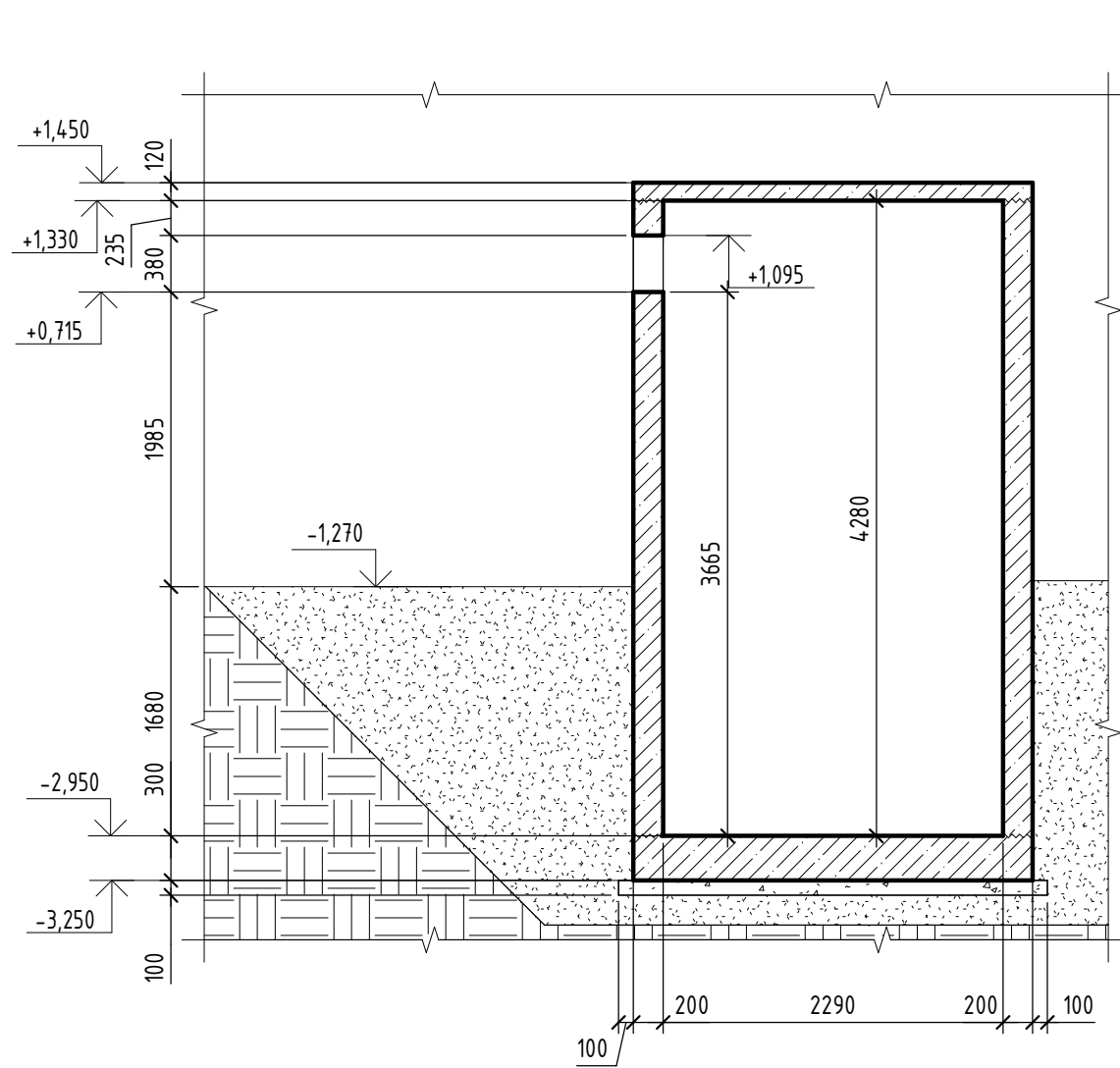
1-1 Опалубка
