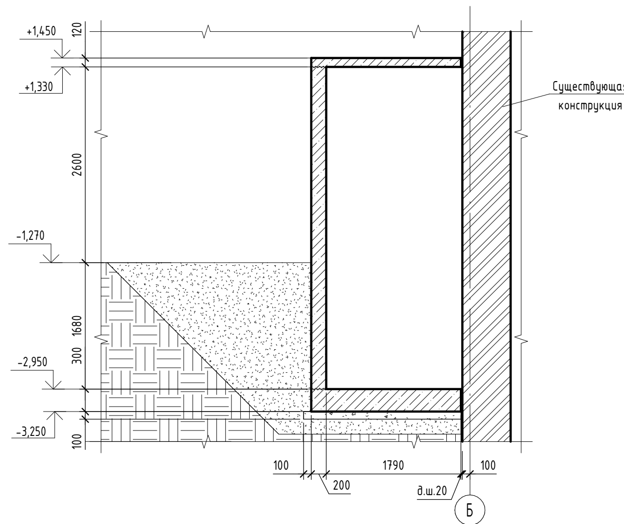
2-2 Опалубка
