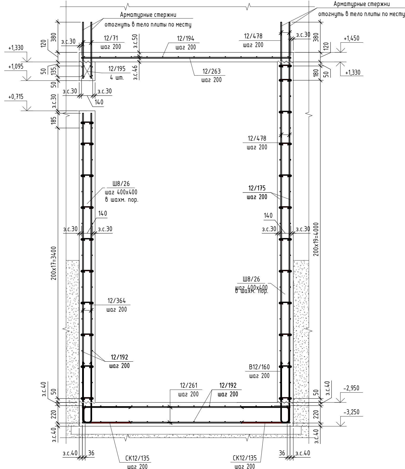
1-1 Армирование
