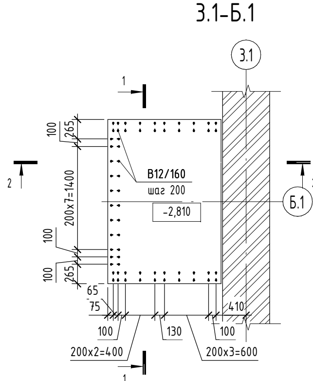
Схема расположения арматурных выпусков фундаментной плиты в/о 3.1-Б.1
